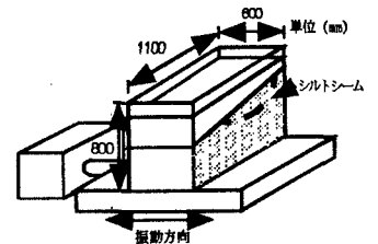
図-1 実験装置の概略図
