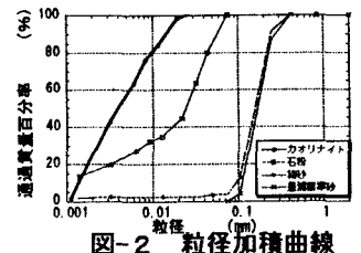
図-2 粒径加積曲線
