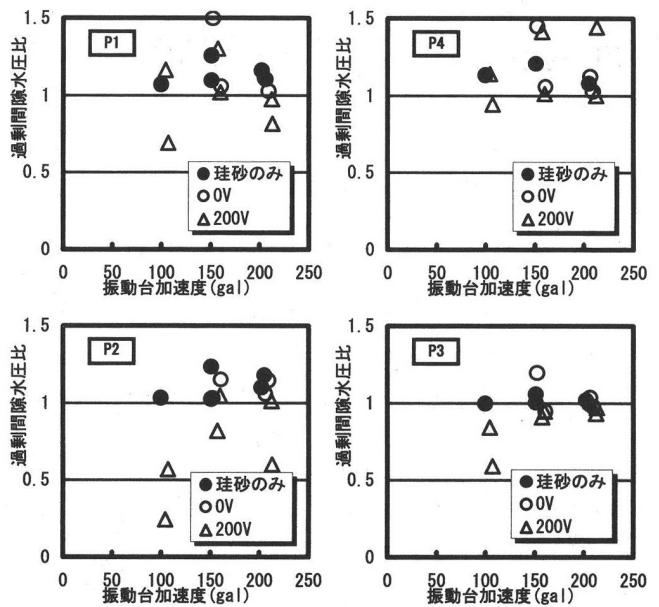
図-2 通电による過剰間隙水圧比の比較
