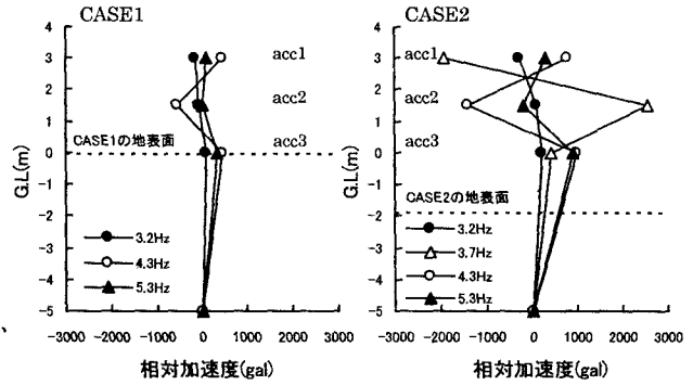
図-3 相対加速度による振動系
