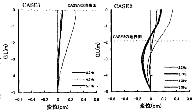
図-5 杭の変位
