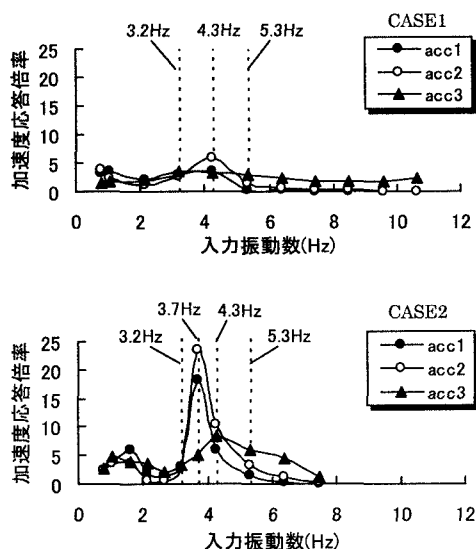
図-2 入力振動数と加速度応答倍率
