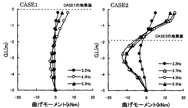
図-4 杭に生じる曲げモーメント
