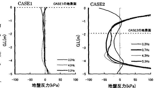
図-6 杭の地盤反力
