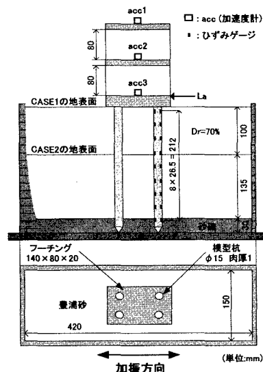
図-1 模型実験装置の概要
