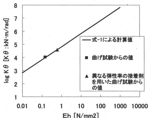
図-5 バネ定数の比較
