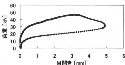
図-4 曲げ試験測定結果
