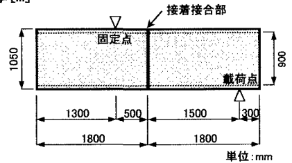
図-2(a) マンホール曲げ試験体
