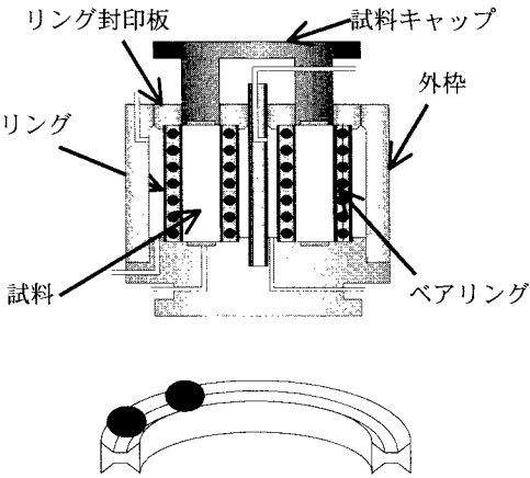
図-1 多段リング式せん断試験機
