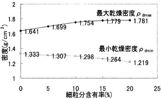
図-2 物理試験結果
