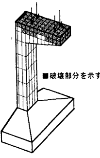
図－8 破壊モード
