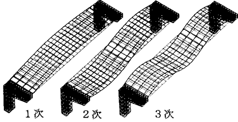
図－5 固有モード形
