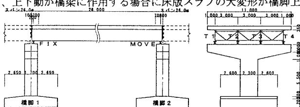
図-1 解析対象橋梁
