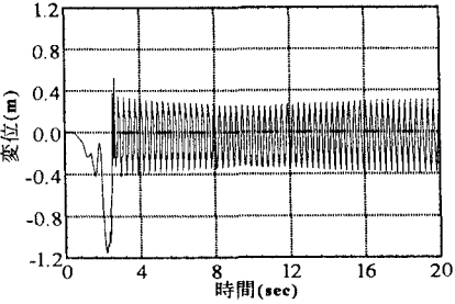
図－6 桁中央部での上下変位の時刻歴
