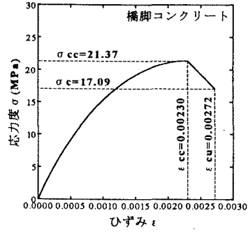
図－4 コンクリートの応力－ひずみ曲線
