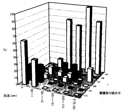
図1-2 段差と支承の損傷の関係
