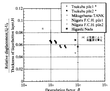
図-7 地盤反力係数の低減率と相対変位（杭と地盤）の液状化層厚による正規化値との関係
