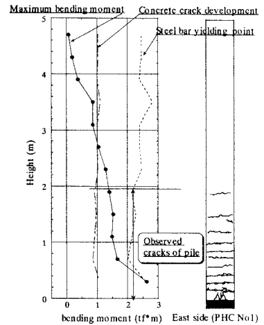
図-5 杭の曲げモーメント分布とクラックの対応
