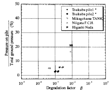
図-6 地盤反力係数の低減率と流動圧比の関係
