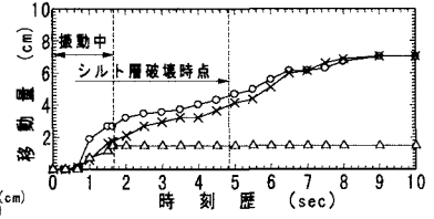
図-5-2 代表点の移動量 (シルトあり)
