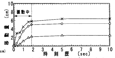
図-5-1 代表点の移動量 (シルトなし)
