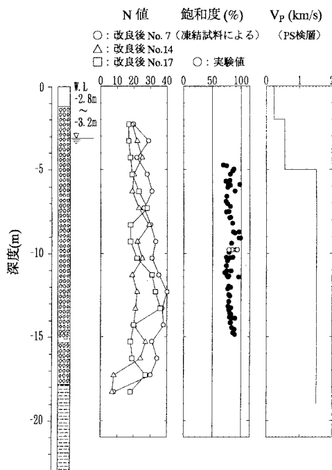
図-1 N値、飽和度、 V_p の関係 1)
