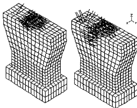
図-5-1 ひび割れ発生状況
