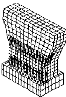
図-6-1 ひび割れ発生状況
