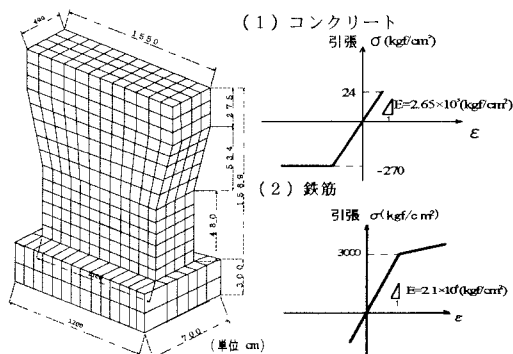
図-3 P 70 のモデル図
