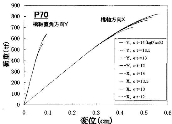
図-8 橋軸方向と橋軸直角方向の荷重と変位
