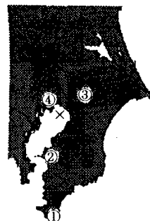
図-1 常時微動観測地点
