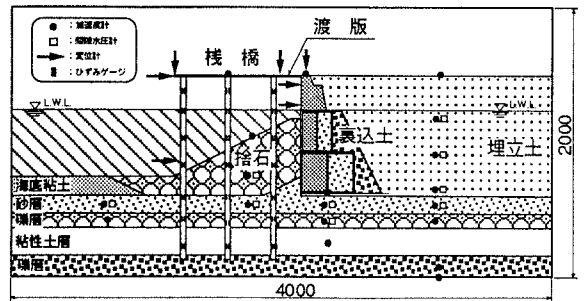
図一 直杭式棧橋振動実験の模型断面
