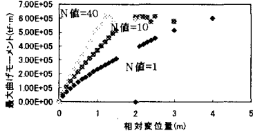
図-10 D=76.2cm の最大曲げモーメント図
