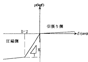
図-6 地盤の非線形性
