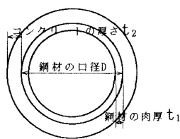
図-3 パイプ断面の形状
