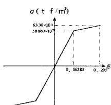
図-4 パイプの非線形性
