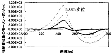
図-8 モーメント分布図
