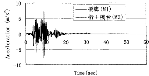
(d) h=0.07 \mu=0.15 の場合
