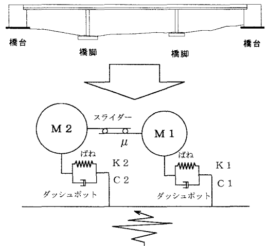
図-1 2 質点系モデル
