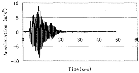
(a) 1 自由度系の場合
