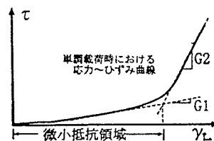
図 2 液状化後の剛性や微小抵抗領域の定義
