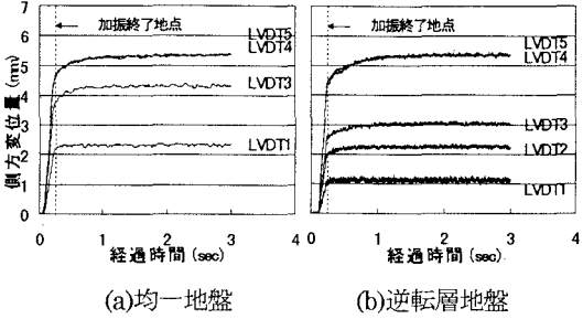
図 4 側方変位量の経時変化
