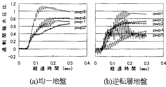
図 3 間隙水圧比の経時変化
