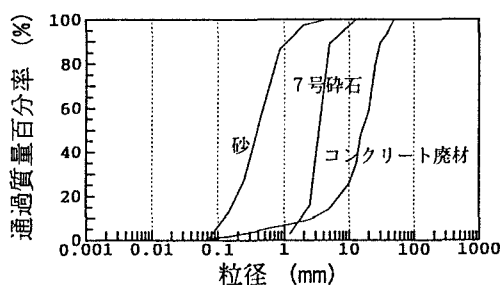
図-2 使用材料の粒径過積曲線
