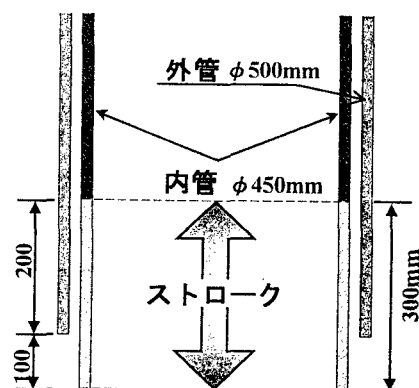
図-1 ケーシング先端の締固め機構
