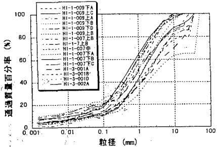
図 1 東灘まさ土の粒度分布
