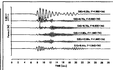
図5 支承に作用する力の時刻歴
