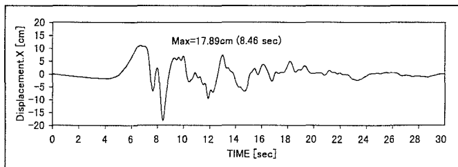
図3 入力波形
