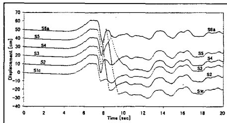
図11 橋桁の応答変位 (S1とS6を分割)
