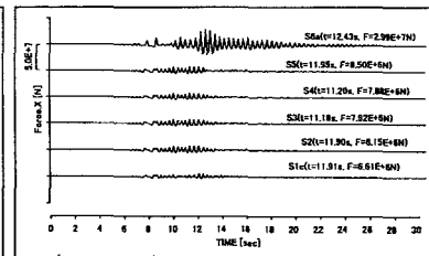
図7 支承に作用する力の時刻歴 (S1, S6 分割)
