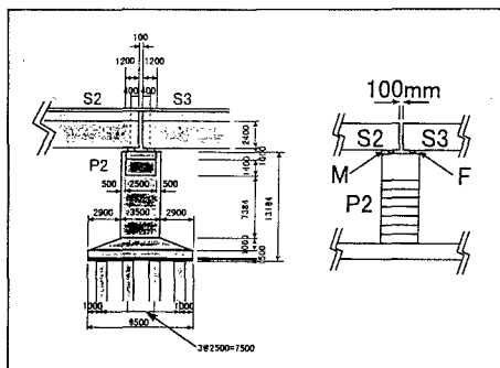
図2 橋脚部分の概寸とその解析モデル
