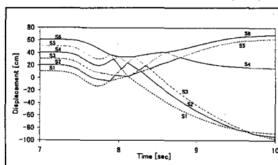
図9 橋桁の応答変位 (図8の拡大図)
