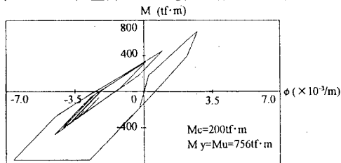
図-7 左柱基部M-φ履歴 (軸力一定)
