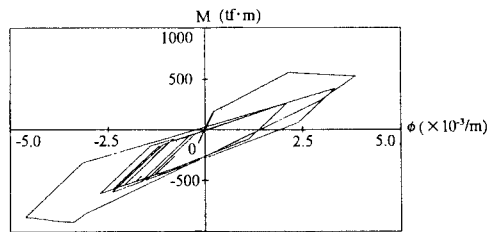
図-8 左柱基部M-φ履歴 (軸力変動考慮)
