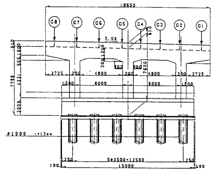
図-1 検討対象の3柱式RCラーメン橋脚
