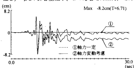
図-3 上部工変位応答波形
