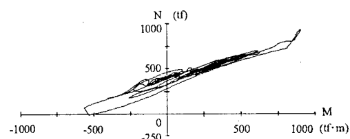
図-6 左柱基部N-M履歴 (軸力変動考慮)
