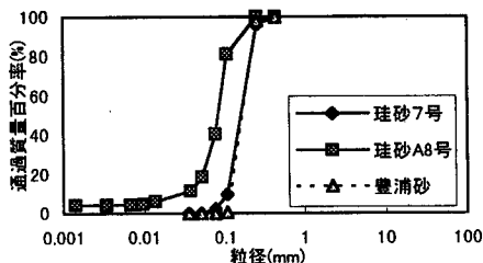
図-1 粒径加積曲線(細砂)
