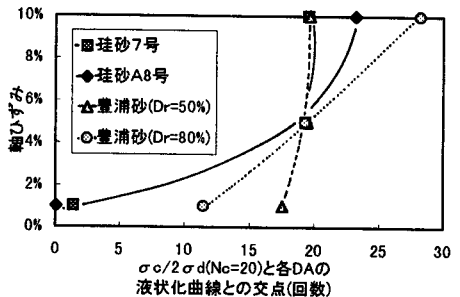
図-6 回数と軸歪みの関係(細砂)
