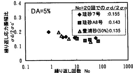
図-3 細砂の液状化抵抗
