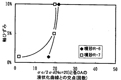
図-7 応力比と軸歪みの関係(噴砂)
