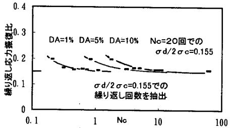
図-5 各DAを液状化判定基準とした珪砂7号の液状化抵抗曲線
