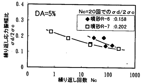
図-4 噴砂の液状化抵抗
