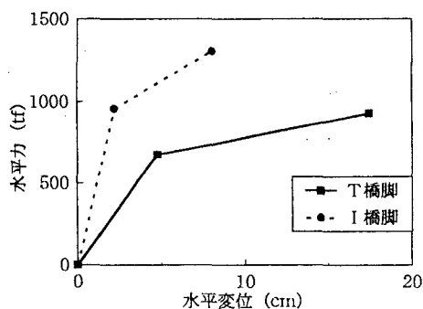
図2 上部構造の慣性力作用位置における水平力～水平変位の関係
