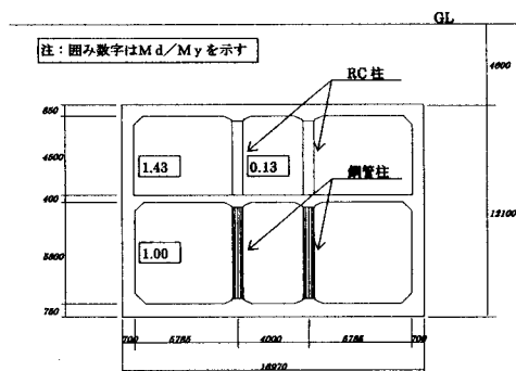
図-4 Md/My の試算例
