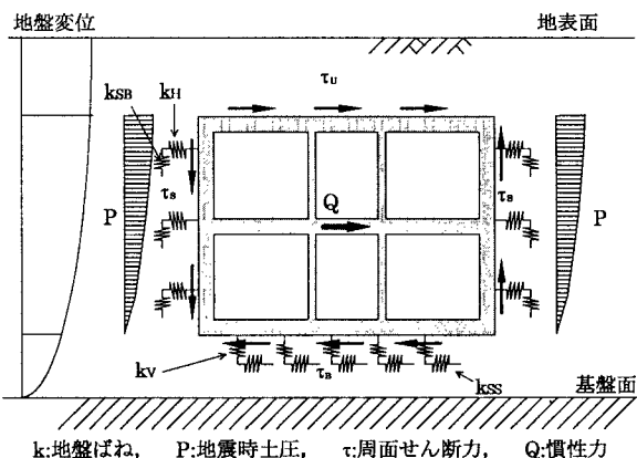
図-3 解析モデルと地震荷重
