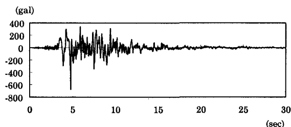
図-1 入力地震動
