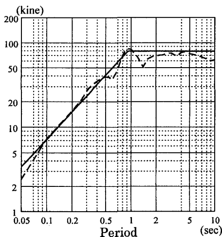
図-2 速度応答スペクトル
