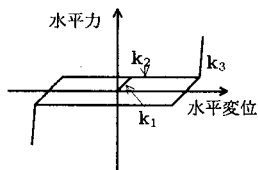
図-2 可動支承モデル
