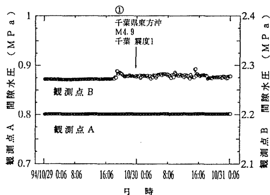
図2 間隙水圧の経時観測結果
