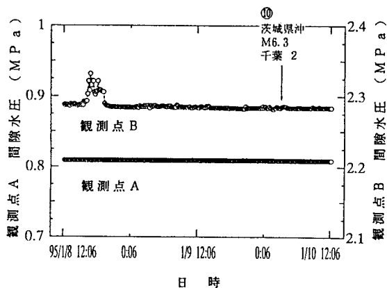
図6 間隙水圧の経時観測結果
