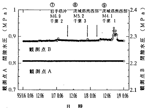
図5 間隙水圧の経時観測結果
