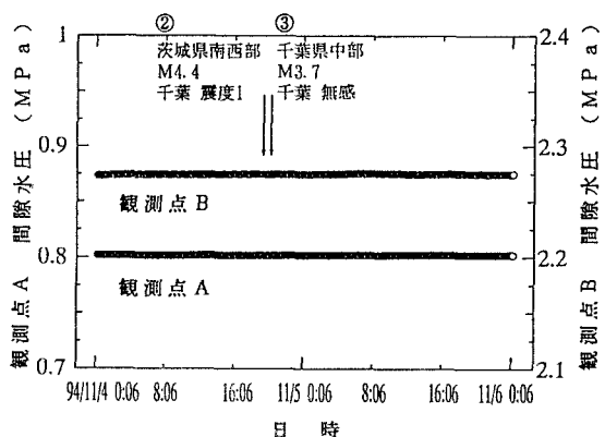
図3 間隙水圧の経時観測結果
