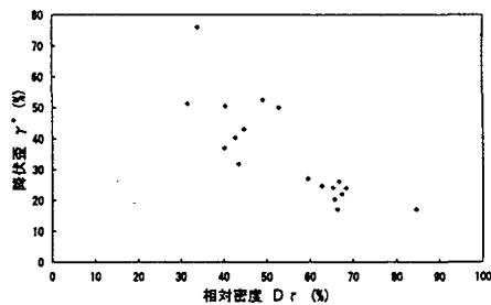
図-5 降伏歪 \gamma^* ～相対密度 D_r 関係(遠州灘砂)
