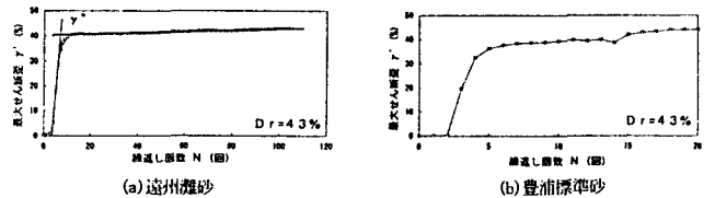
図-4 最大せん断歪 \gamma^* ～繰返し回数 N 関係
