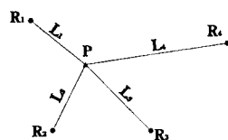
図-1 Method1 の概念図
