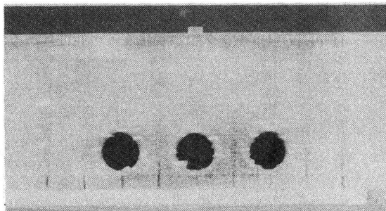
写真1 3本併設トンネル模型振動実験
