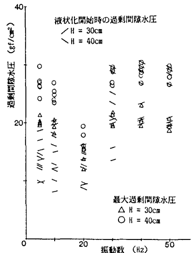
図-3 振動数-過剰間隙水圧
