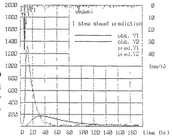
図-4 流出予測
