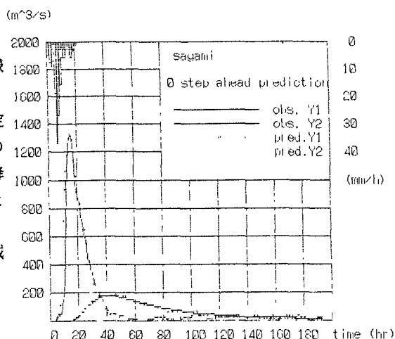
図-1 流出解析
