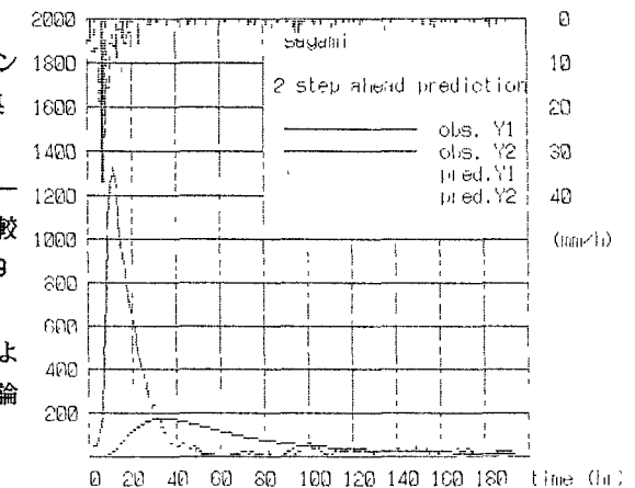
図-5 流出予測
