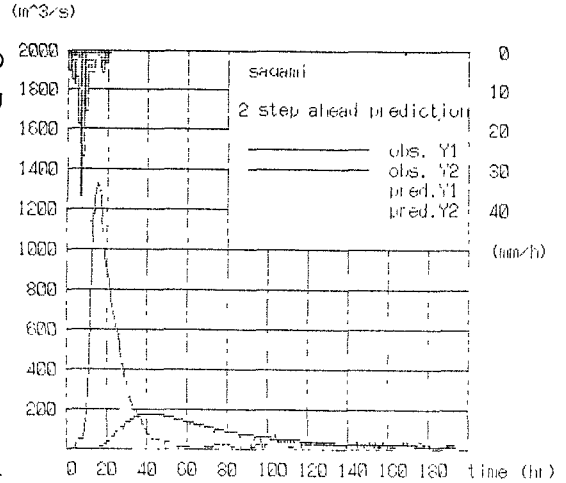
図-3 流出予測
