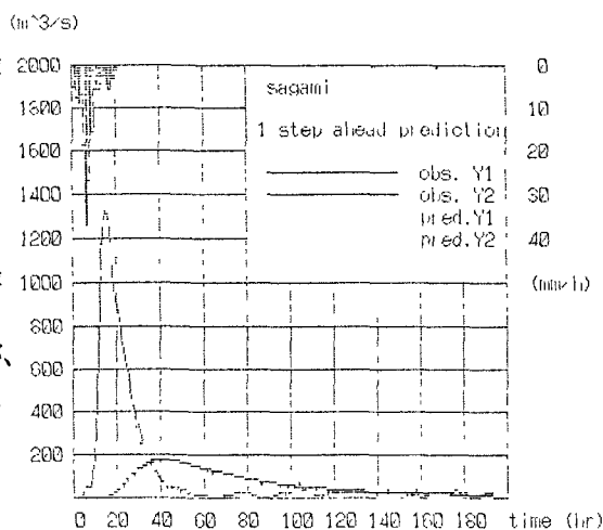
図-2 流出予測
