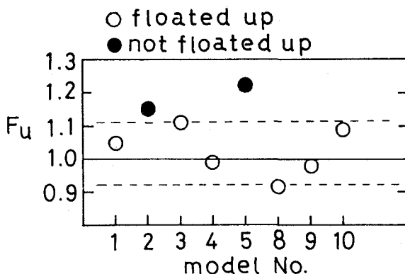
図3. 半地下構造物模型が浮上り始めるときの浮上の安全率
