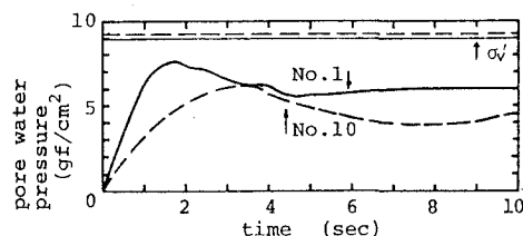
図4. 模型No.1とNo.10の半地下構造物模型の底面に作用する間隙水圧の比較
