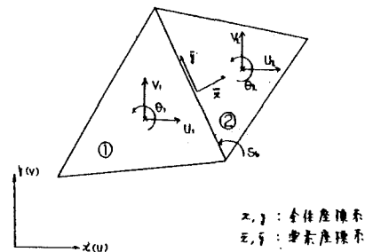
図-1 隣接する新しい三角形要素
