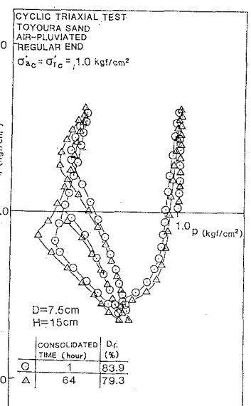
図-6. 有効応力経路 (圧密時間の影響)
