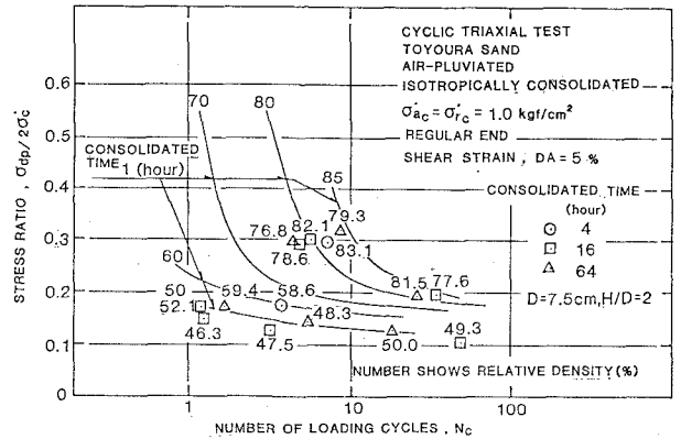
図-3. 応力比へ繰返し回数(圧密時間の影響)
