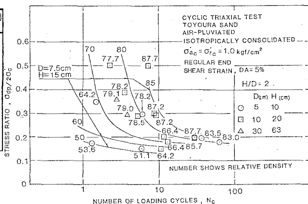
図-1. 応力比～繰返し回数（直径の影響）
