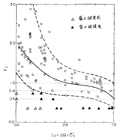
図-4 F_L と 過剰間隙水圧比の関係
