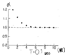
図-5 A波に対する試算例
