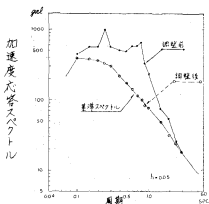
図-6 B波に対する試算例
