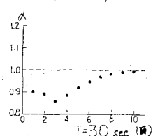
図-7 繰り返し回数によるスペクトル比( \alpha )の収れん状況 (A波)
