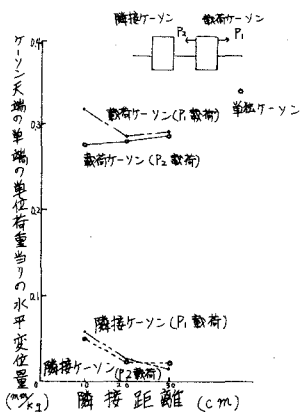
図-1 隣接距離と静的載荷によるゲルソン変位の関係
