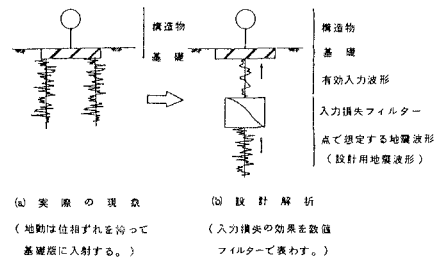
図-2 地震波の入力機構
