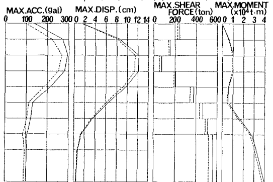
図-7 最大応答結果 (1968 千代田 (H) EW)
