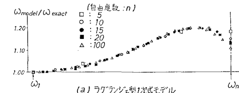
(a) ラグランジュ型1次モデル
