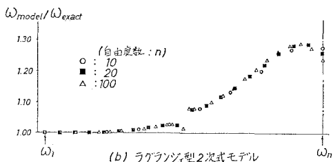
(b) ラグランジュ型2次モデル
