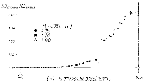
(c) ラグランジュ型3次モデル
