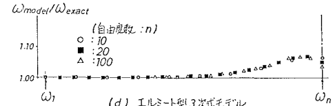
図-5 各モデルの固有振動数分布形状
