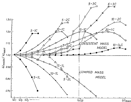
図-4 各モデルの固有振動数の理論解との比
