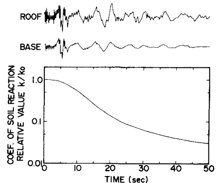
Fig. 6 地盤反力係数の時間的な変化
