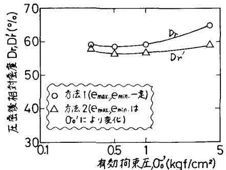
図3. \sigma'_0 の増加に伴う D_r , D_r' の変動
