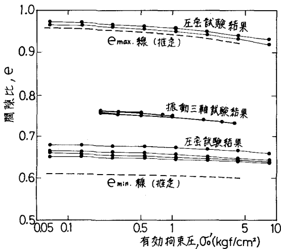
図2. \sigma'_0 と e の関係
