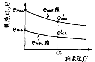
図1. e_{max} , e_{min} と \sigma'_0 の関係
