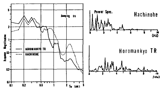
図-4 八戸及び隈満橋TRのスペクトル特性。
