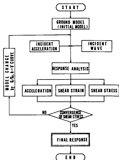
図-1 応答計算流れ図
