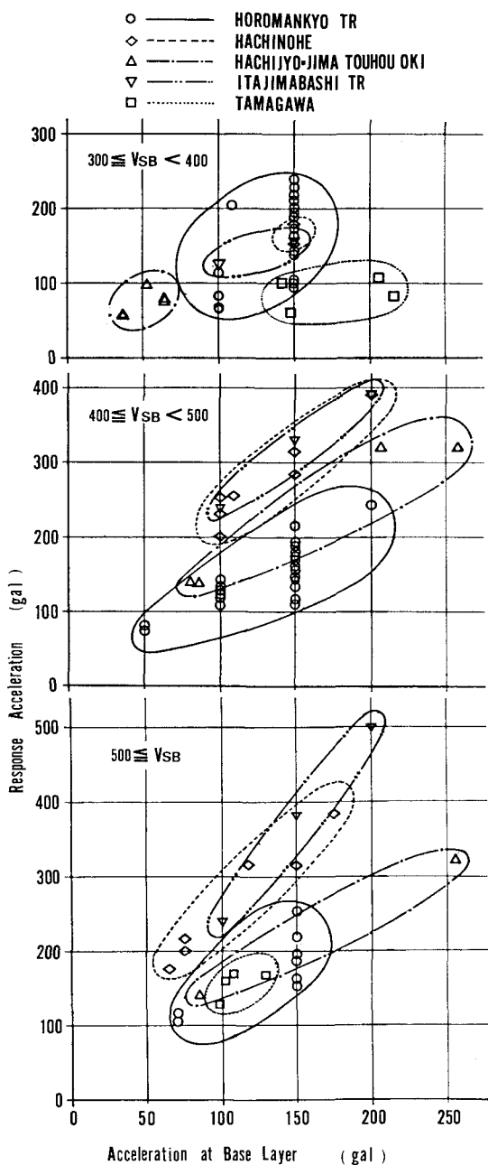
図-2 基盤波速度別の基盤加速度と地表応答加速度との関係。
