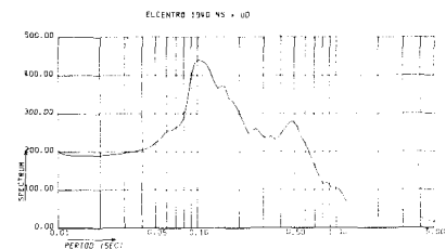
図-5 水平成分波形の加速度応答スペクトル(エルセントロ波水平上下動入力)
