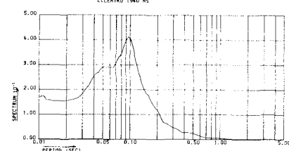
図-6 ロッキング成分波形の加速度応答スペクトル(エルセントロ波水平動入力)
