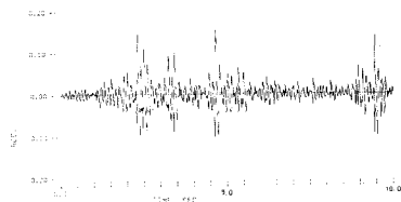
図-2 ロッキング成分の応答加速度波形(エルセントロ波水平動入力)
