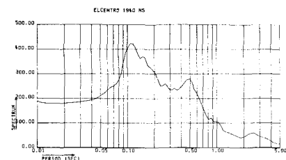
図-4 水平成分波形の加速度応答スペクトル(エルセントロ波水平動入力)
