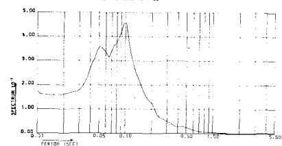
図-7 ロッキング成分波形の加速度応答スペクトル(エルセントロ波水平上下動入力)
