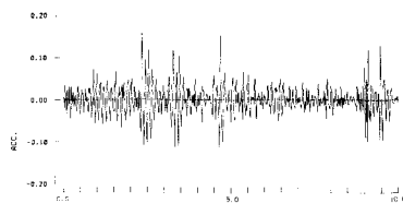
図-3 ロッキング成分の応答加速度波形(エルセントロ波水平上下動入力)
