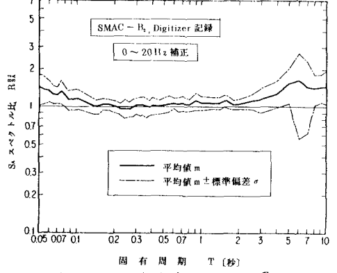
(c) 0~20 Hzまで補正を施した場合
