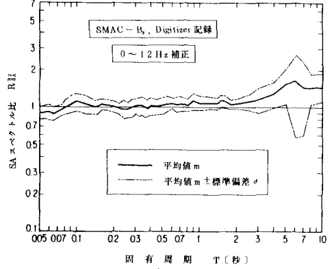
(b) 0~12 Hzまで補正を施した場合
