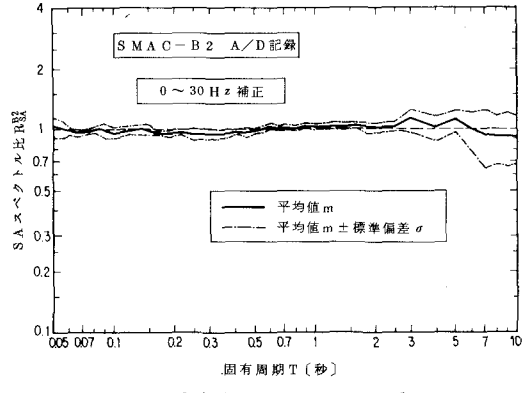
(c) 0~30 Hzまで補正を施した場合
