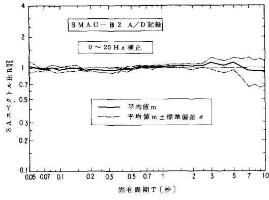
(b) 0~20 Hzまで補正を施した場合
