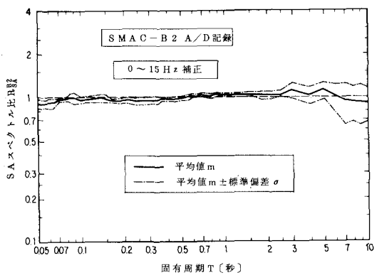
(a) 0~15 Hzまで補正を施した場合
