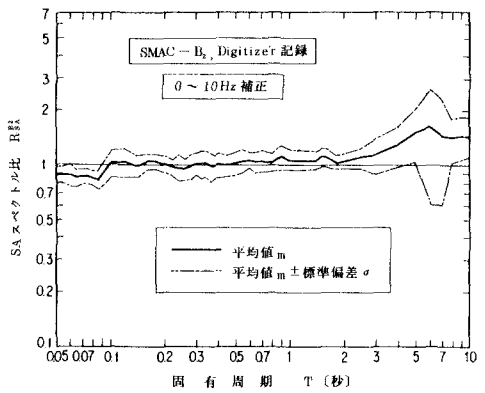
(a) 0~10 Hzまで補正を施した場合
