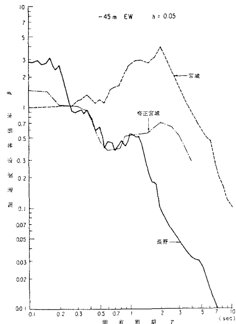
図-4 全震源地地震記録の応答スペクトルの修正(地下45m, EW成分)
