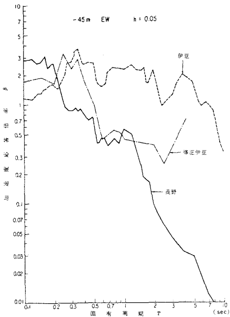
図-3 全震源地地震記録の応答スペクトルの修正(地下45m, EW成分)
