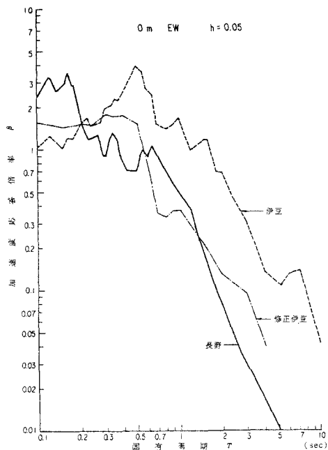
図-2 全震源地地震記録の応答スペクトルの修正(地表面, EW成分)
