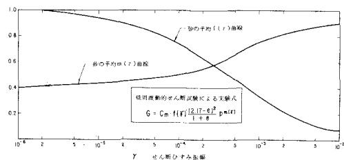
図-3 簡易評価法のひずみの関数
