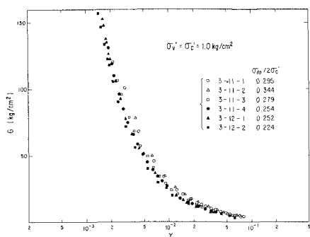
図-1 G ~ γ 曲線
