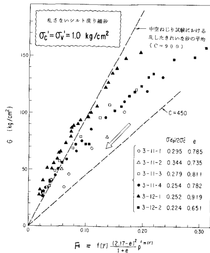
図-4 G 実測値と簡易評価法による推定値
