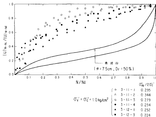
図-2 間隙水圧と載荷回数
