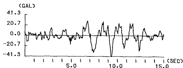
(a) 静内橋地震動加速度記録
