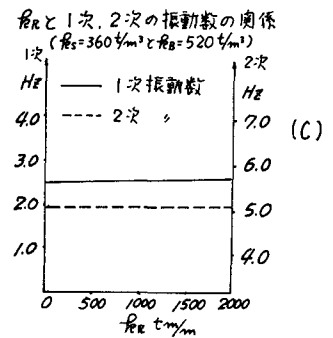
図-6 地盤のバネと振動数の関係
