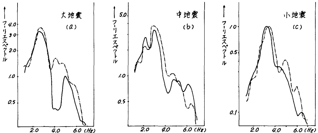
図-7 橋脚上のフリエスペクトル(—実録加速度記録, ---モデルから計算された応答加速度)
