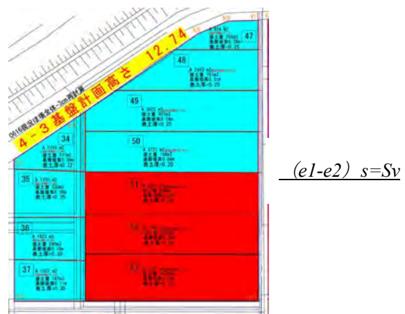
図 10 セグメント毎の切盛土量算出結果
