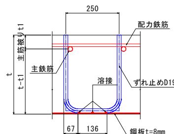
図-2 ずれ止め筋詳細図
