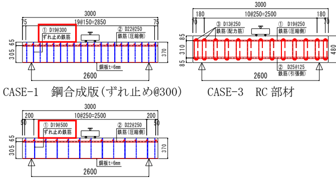
図-3 供試体形状図
